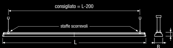
Posizione di installazione apparecchio 2x
