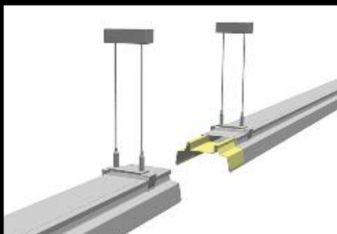
staffa rapida di connessione lineare
