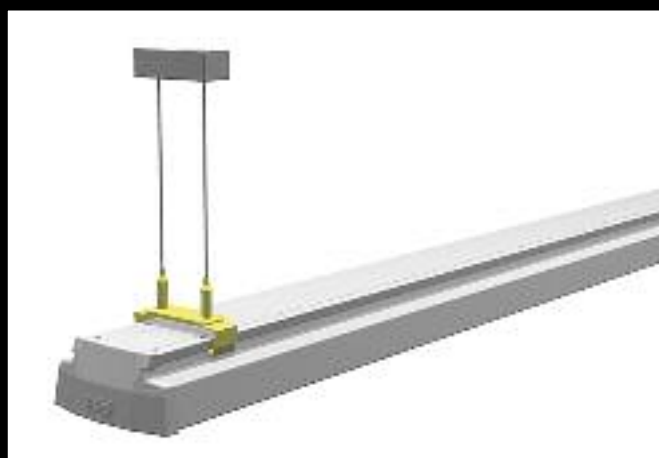
sistema di sospensioni a interasse di installazione variabile con staffa scorrevole. Interasse consigliato: L-200 mm
